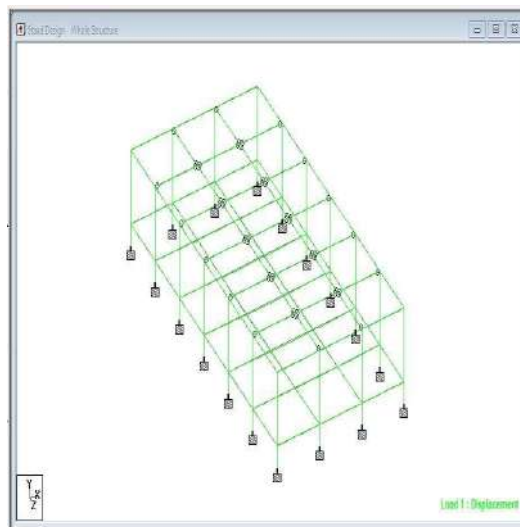
Fig. 2.1.1 MODELING
