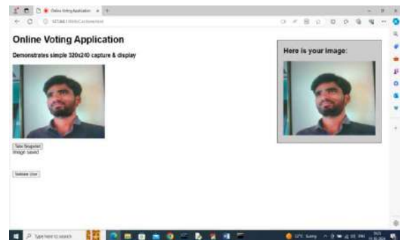
Fig.4.15 Take Snapshot
