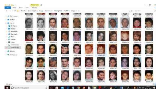
Fig.5.1 Dataset
